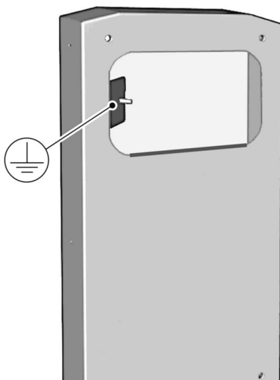
Punto de puesta a tierra
